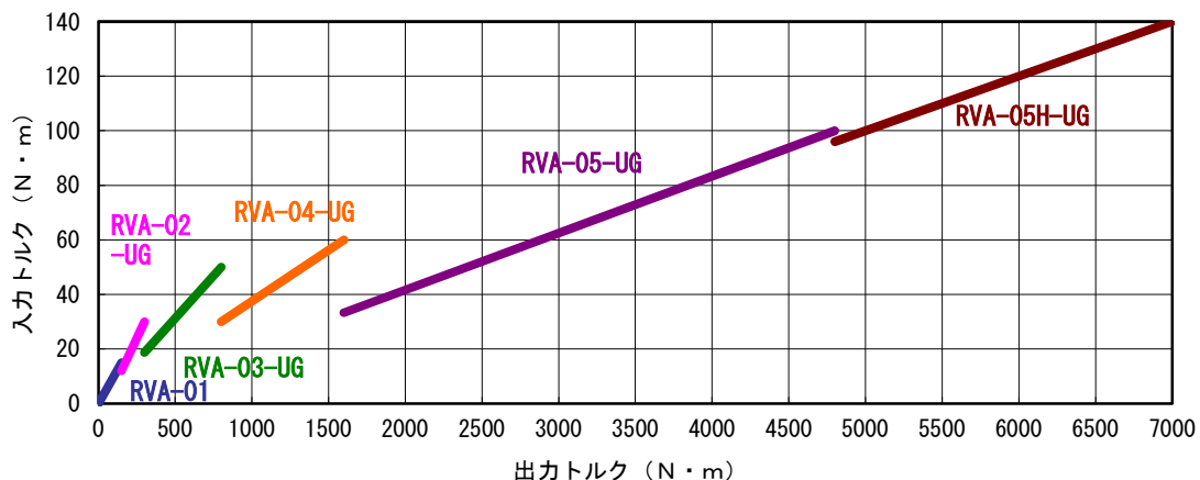
トルク線図
