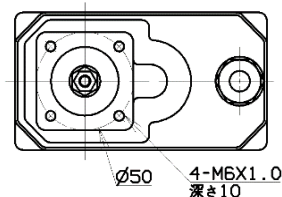
外観図
