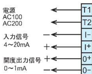
結線図
